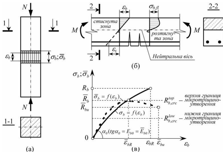
Рис. 1. Напружено-деформований стан нормальних перерізів бетонного й залізобетонного елементів: (а) однорідний НДС за осового стиску; (б) неоднорідний НДС згину; (в) діаграми деформування бетону \sigma_b = f(\varepsilon_b) і \bar{\sigma}_b = f(\varepsilon_b) відповідно у «м'якому» і «жорсткому» режимах короточасного осового стиску
