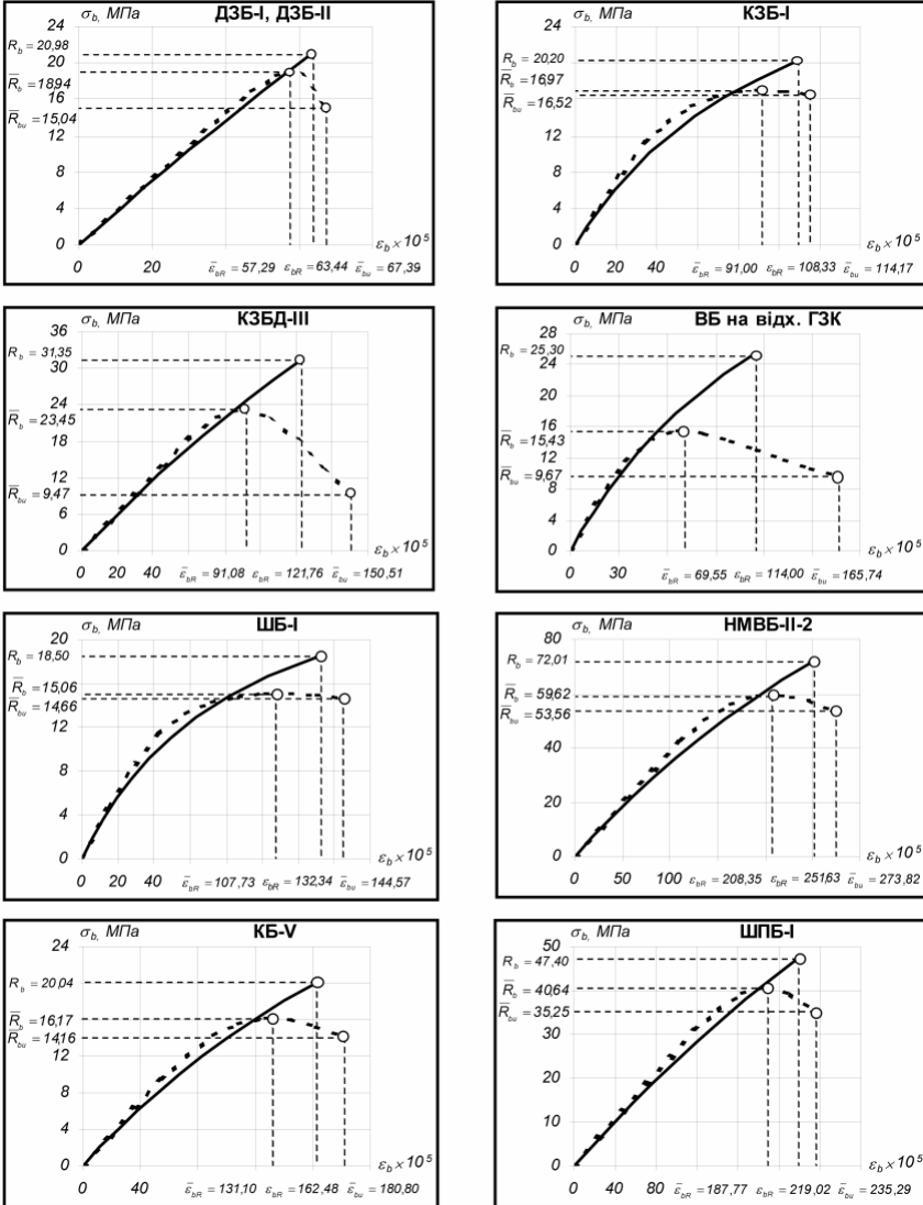
Рис. 3. Приклади трансформування діаграм поздовжнього деформування різних видів бетону за короточасного осового стиску (позначення ті ж самі, що у Табл.і 2 і рис. 2)
