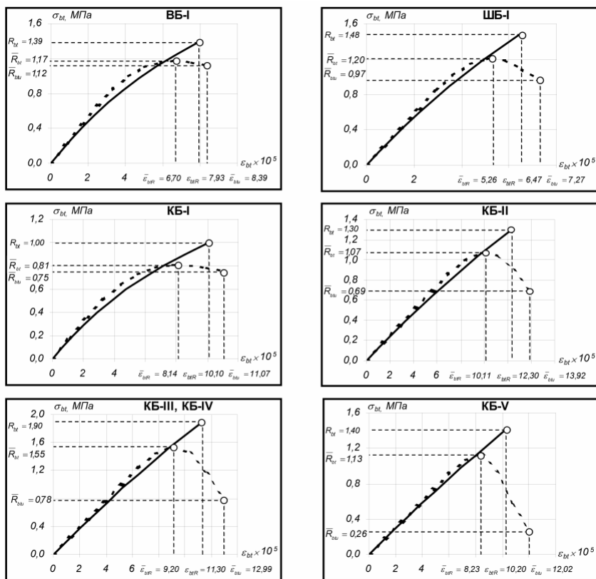
Рис. 4. Приклади трансформування діаграм поздовжнього деформування різних видів бетону за короткочасного осевого розтягу (позначення ті ж самі, що у Табл. 2 і рис. 2)
