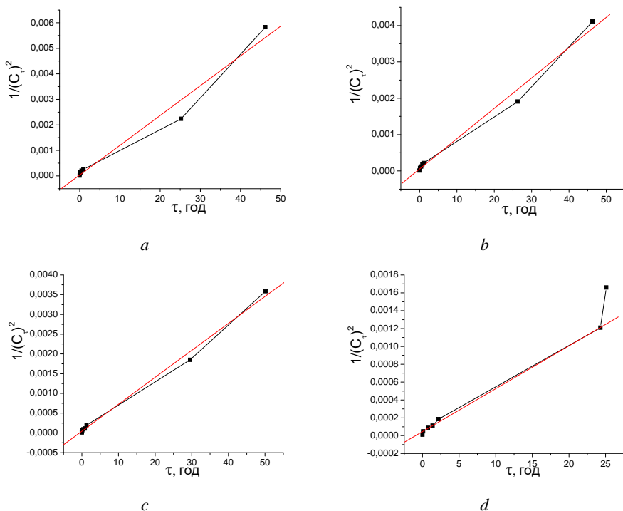
Рис. 3. Зміна квадрата оберненої концентрації іонів \text{Fe}^{3+} з часом: а) реакційна суміш 4; б) реакційна суміш 5; в) реакційна суміш 6; г) реакційна суміш 7.
