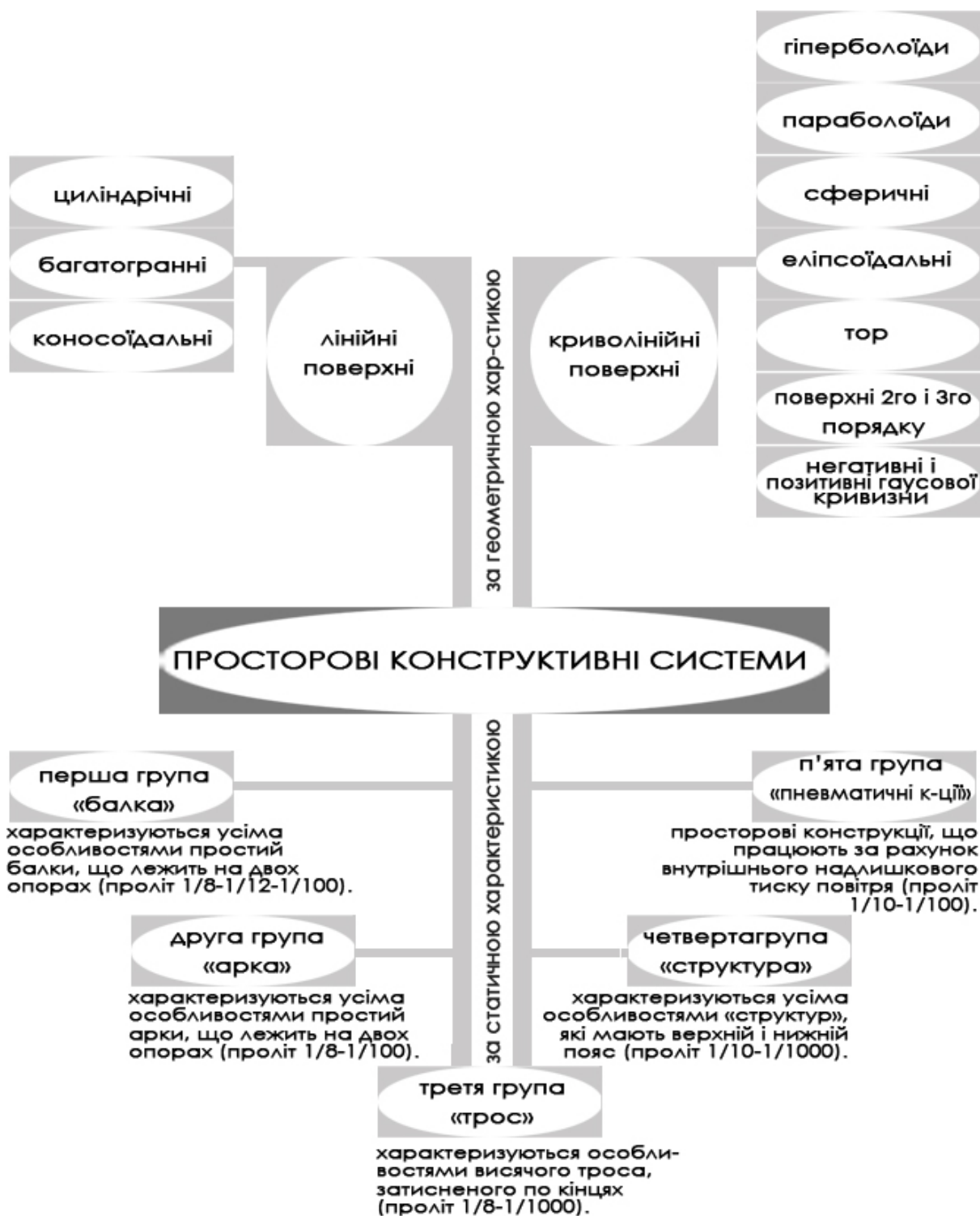
Рис.1.2 Класифікація просторових конструктивних систем
