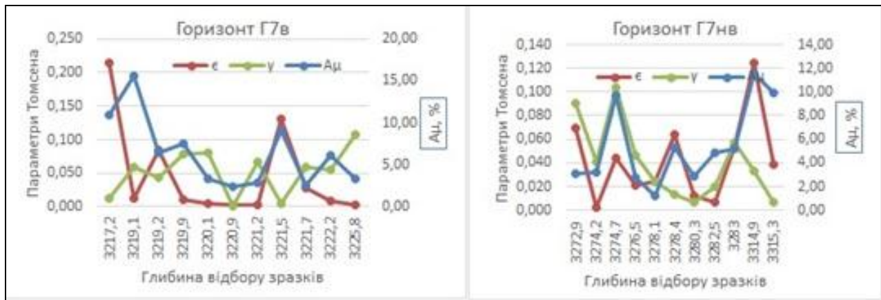
Рис. 6. Графіки залежностей параметрів Томсена та інтегрального акустичного коефіцієнта анізотропії для зразків продуктивних горизонтів Руновщинської площі; а – горизонт Г7в, б – горизонт Г7нв
