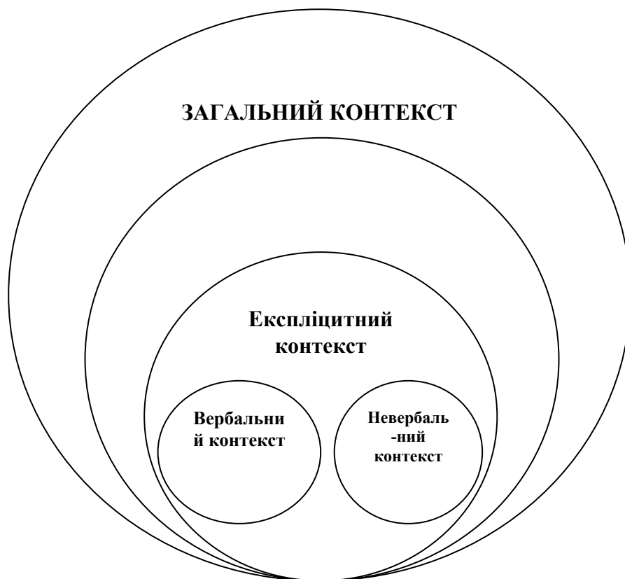
Рис. 1. Контекстуально-динамічний аналіз
