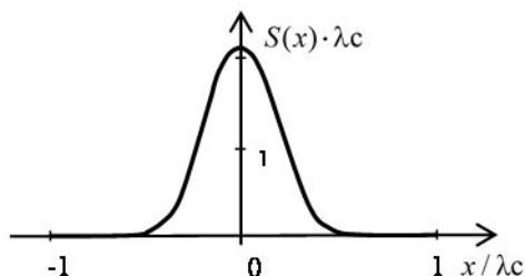
Рис. 3. Весовая функция фазокорректированного «50% Гауссова фильтра»
