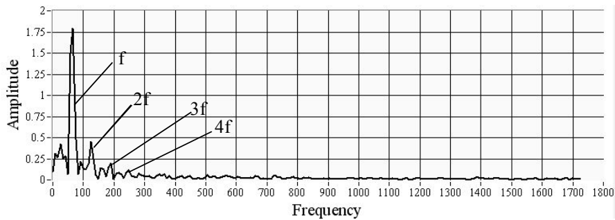
Рис. 7. Спектрограмма оцифрованной профилограммы поверхности образца № 5.1
