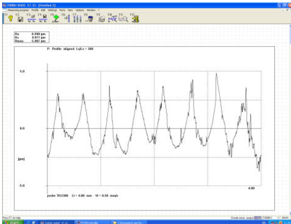
Рис. 5. Профилограмма поверхности образца № 5.1 при lt = 4,8 мм (станция Т8000)
