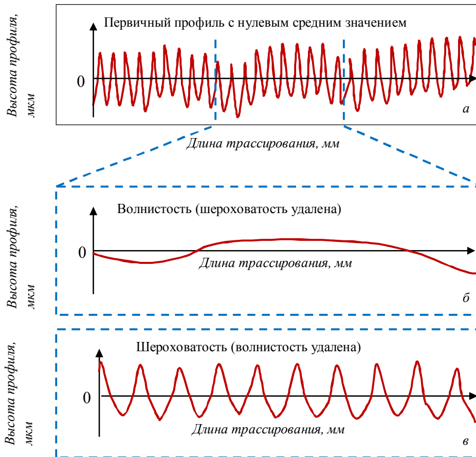
Рис.2. Фильтрация сигнала первичного профиля (а) с выделением сигнала волнистости (б) и шероховатости (в) (не содержит формы и отклонения формы)
