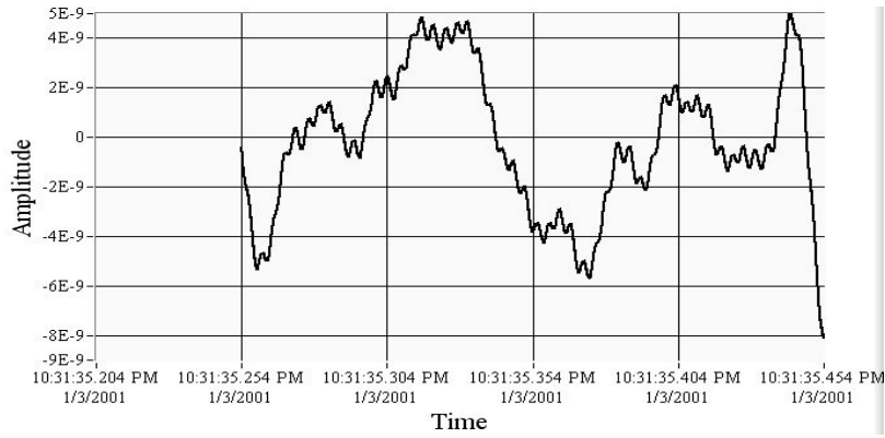
Рис. 6. Временной сигнал виброперемещения при плоском фрезеровании образца № 5.1 (вибродатчик AP2019 расположен на заготовке в направлении оси X станка мод. 500V/5)
