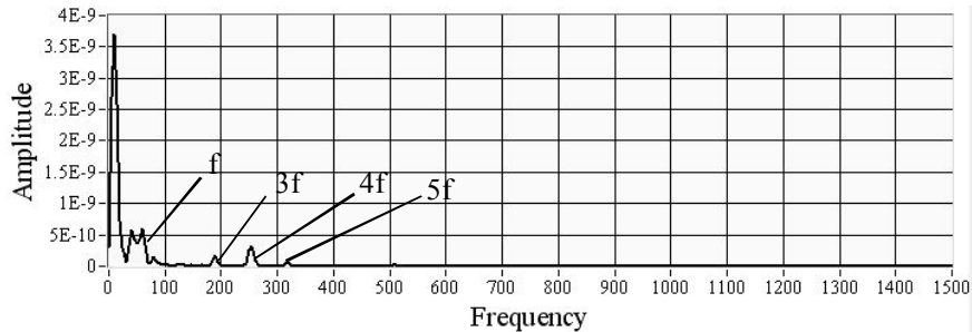
Рис. 8. Спектрограмма сигнала виброперемещения при обработке участка образца № 5.1
