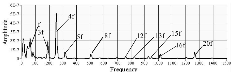
Рис. 10. Спектр сигнала виброскорости
