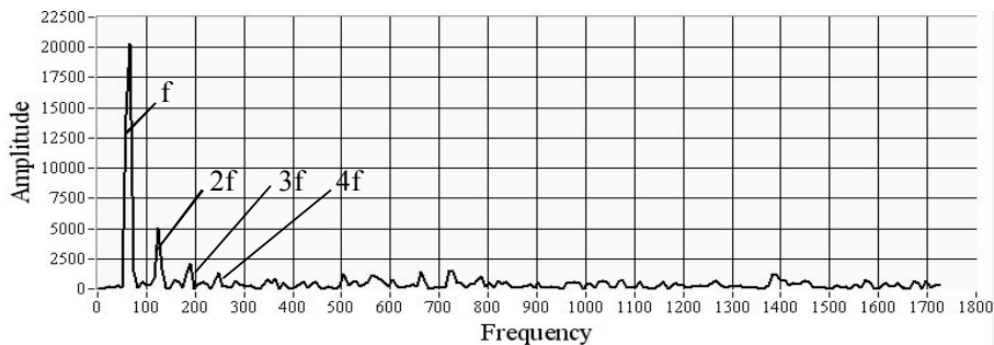
Рис. 9. Спектр скоростной характеристики профилограммы
