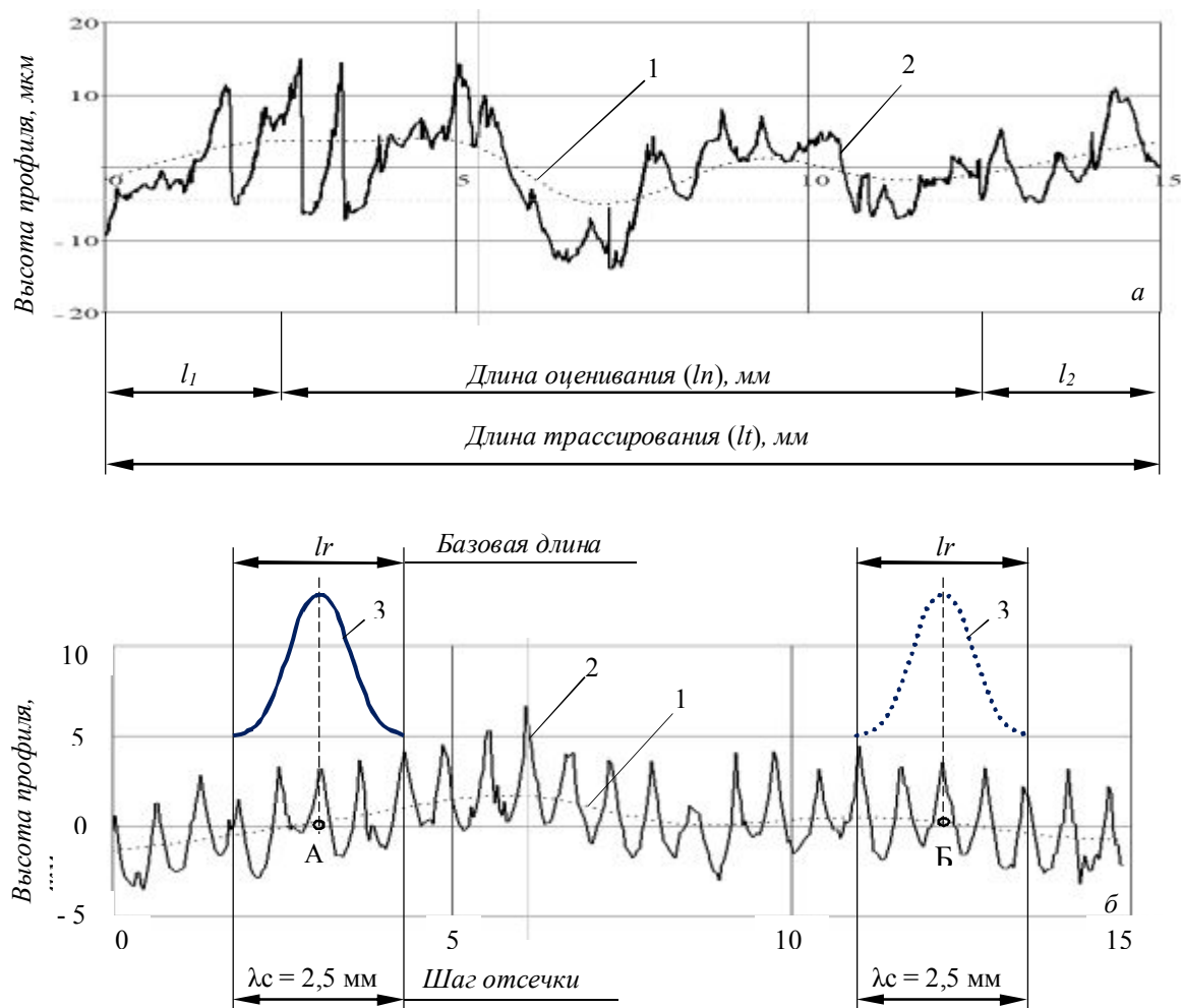
Рис. 4. Построение волнограмм поверхности (1) на основе оцифровки первичной профилограммы (2) с применением функции сглаживания Гаусса (3) для образцов № 2.1 (а) и № 5.1 (б)
