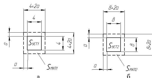
Рисунок 2 – Электронные компоненты с размерами a - 4 \times 4 \text{ мм} и б - 8 \times 8 \text{ мм}
