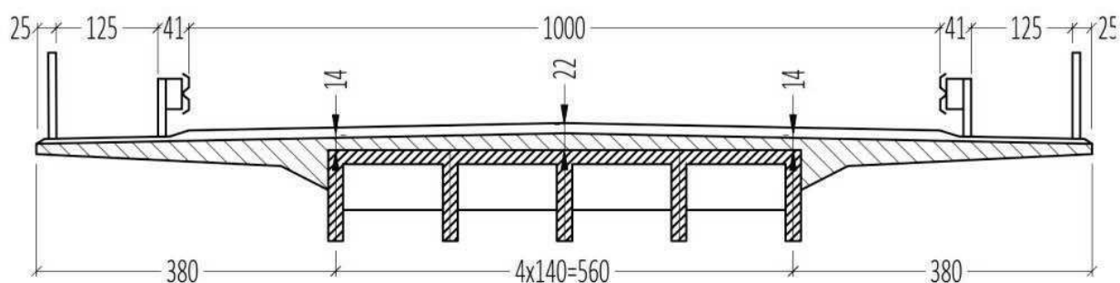
Рис. 3. Міст через р. Прутець-Яблунецький на а/д Мукачеве-Львів в с. Татарів Івано-Франківської області. Розширення прольотної будови монолітною залізобетонною накладною плитою
