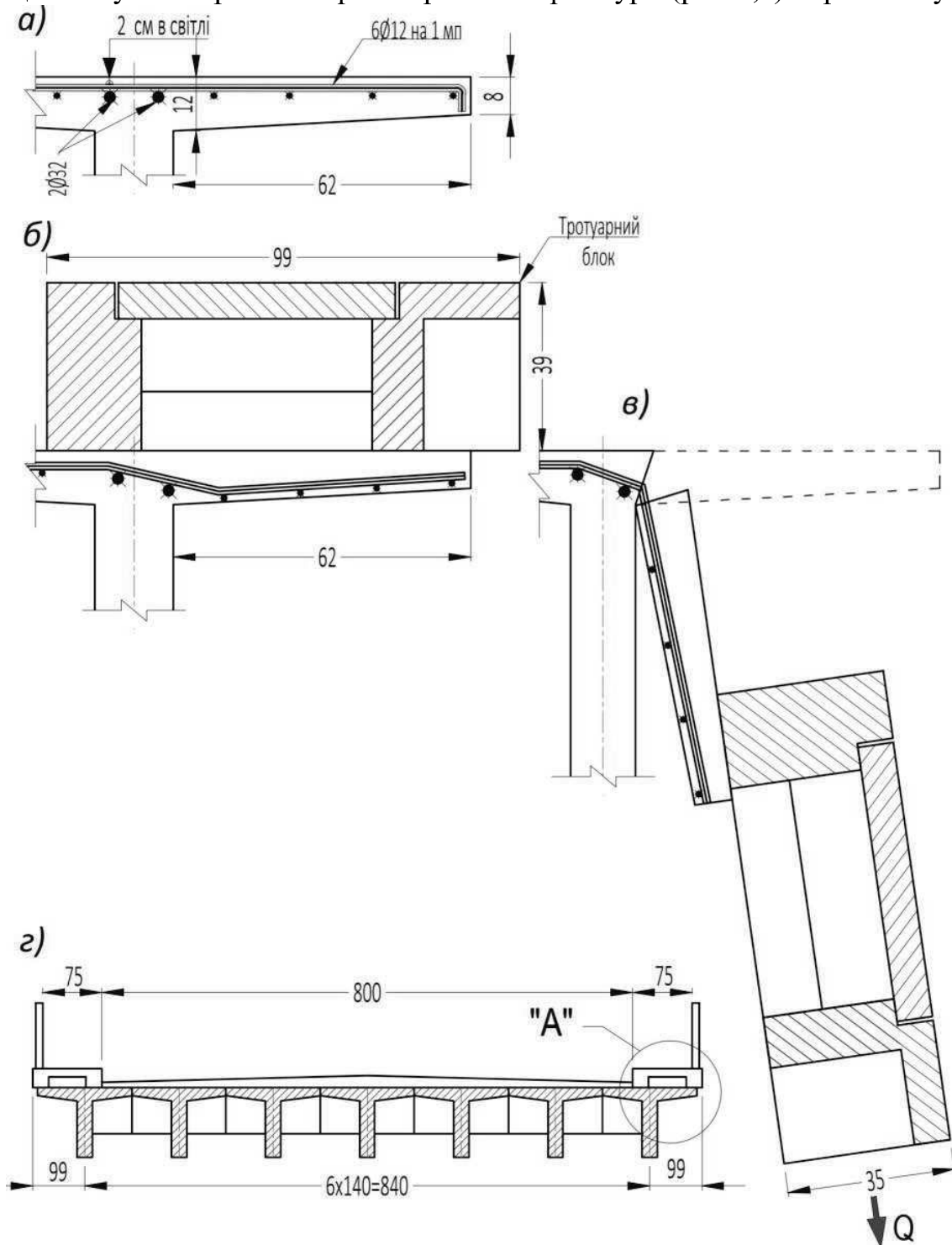
Рис. 1. Міст через р. Іква на автодорозі Київ-Чоп у м. Дубно. Злам тротуарної консолі і обвалення тротуарних конструкцій а – проектне армування консолі крайньої балки за ТП вип. Вип. 56; б – фактичне розташування арматури на консолі і розташування тротуарних конструкцій(деталь «А»); в – злам консолі і обвалення тротуарних конструкцій; г – схема поперечного перерізу прольотної будови з балок за ТП вип. 56.
