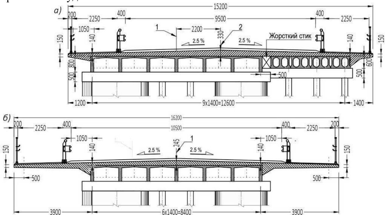
Рис. 4. Міст через р. Іква по вул. Замковій у м. Дубно на а/д Доманське (на Брест) – Мамалига (на Кишинів)
