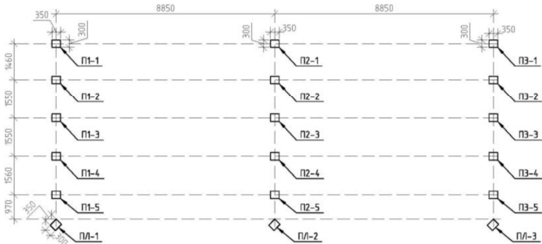
Рис. 3. Маркування паль (стояків) опор моста
