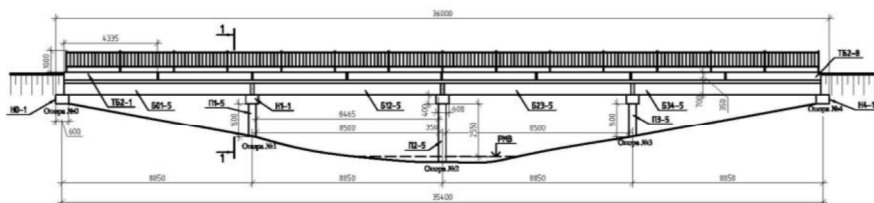
Рис. 2. Поздовжня схема моста
