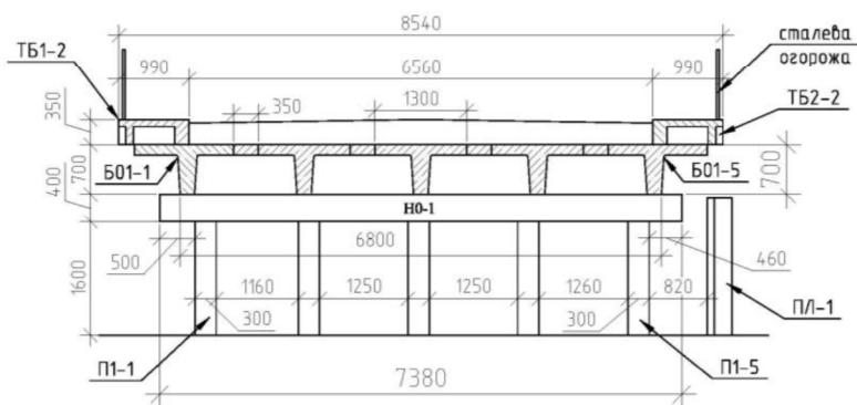
Рис. 1. Поперечна схема моста
