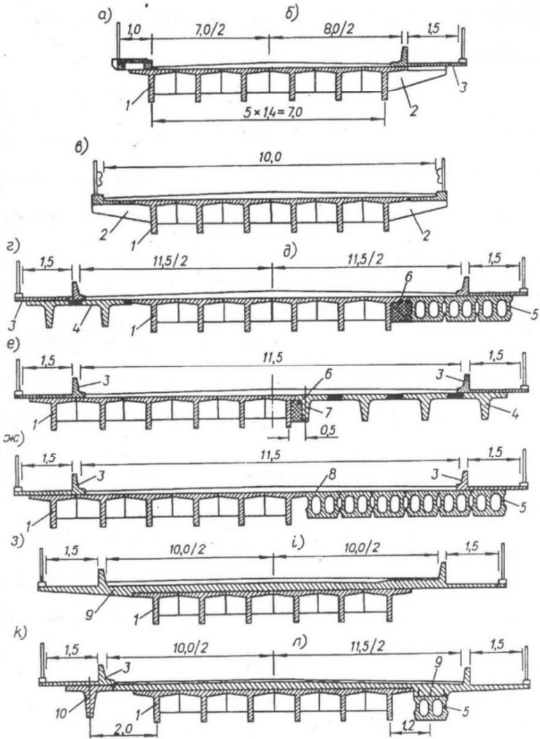
Рис.1. Базові способи розширення ребристих прольотних будов:
