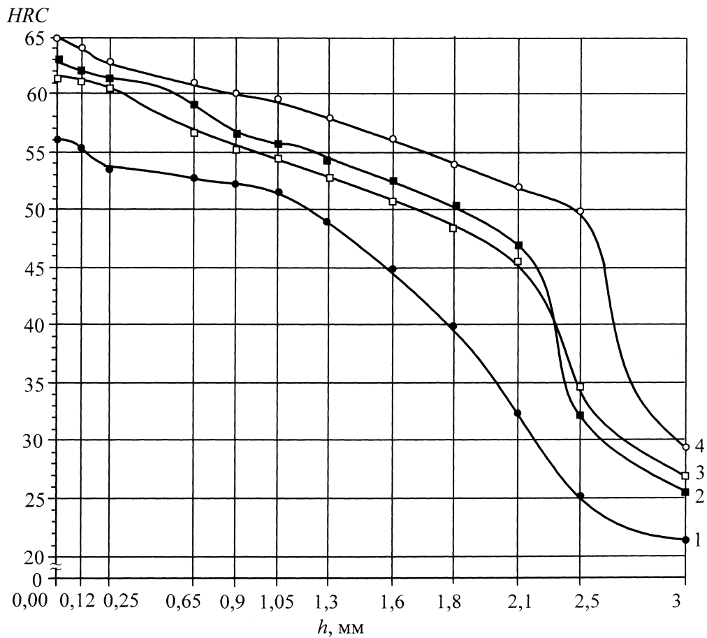
1 – плавка №11 (друге гартування 1083K, відпуск 468K); 2 – плавка №11 (друге гартування 1123K, відпуск 433K); 3 – плавка №22 (відстає азотом при цементації, друге гартування 1083K, відпуск 438K); 4 – плавка №22 (друге гартування 1123K, відпуск 372K)
