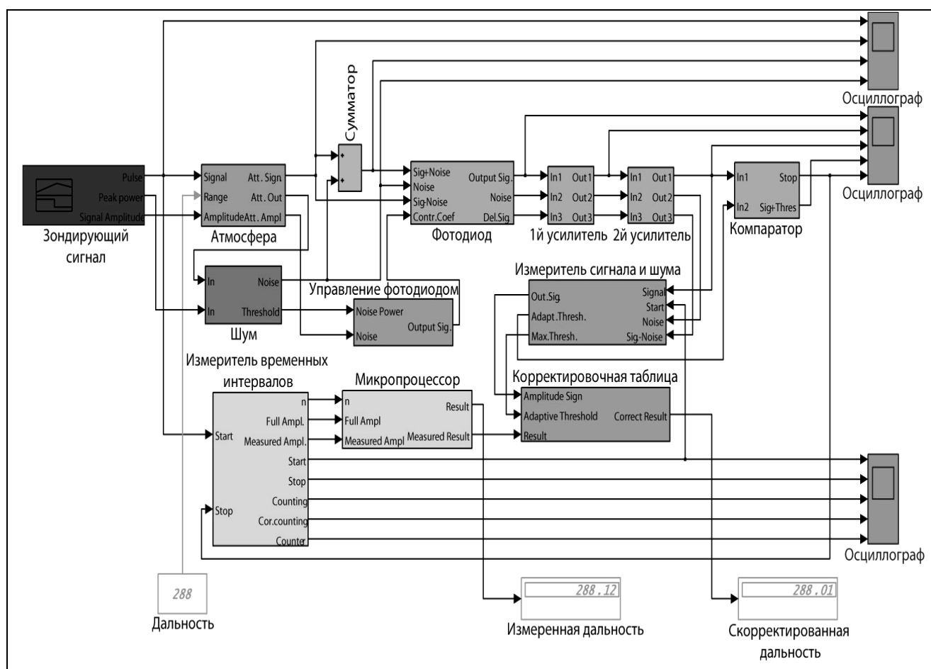
Рис.1. Имитационная модель ЛДУ
