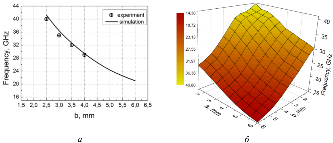
Рис. 3. Зависимости плазменной частоты f_p от периодов проволочной структуры
