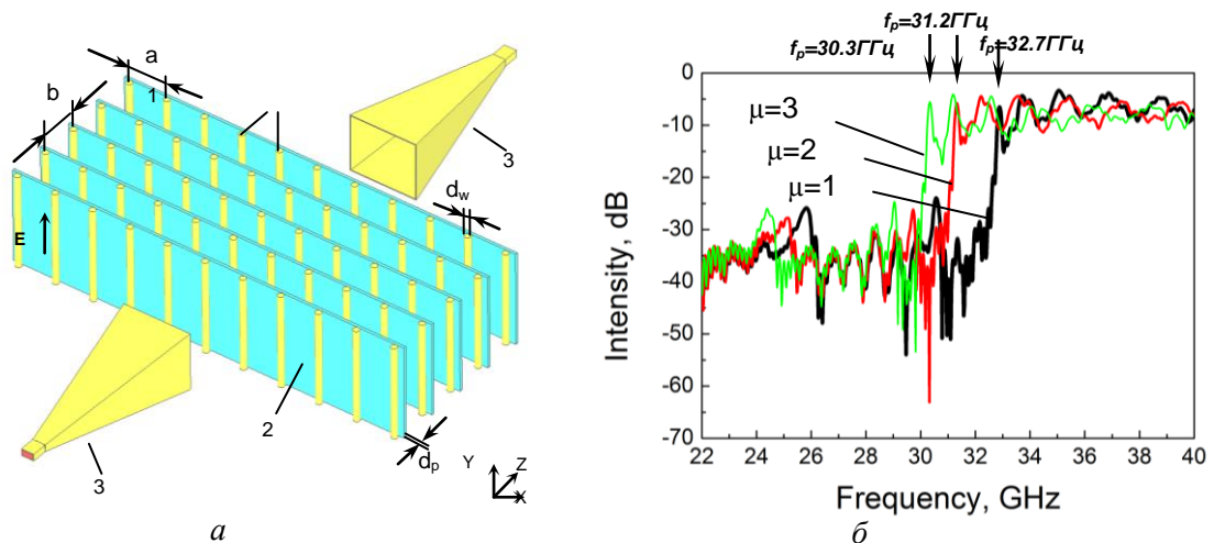
Рис. 4. a – Общий вид проволочной структуры: 1 – медные проволочки; 2 – магнитная подложка; 3 – рупоры; б – спектральные характеристики структуры для различных значений параметра \mu
