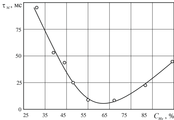
Рисунок 2 – Залежність часу затримки спалахування \tau_{зс} від вмісту Mg у частинках C_{Mg} .
