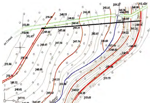
Рис. 2. Фрагмент водосховища № 7
