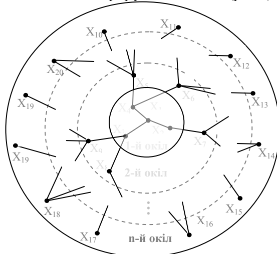
Рис. 1. Околи та межі вузлів графу рухомої системи радіозв'язку
