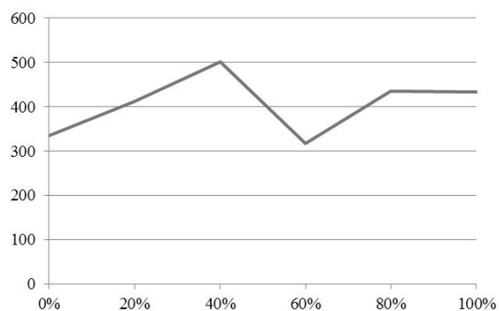
Рис. 6. Зависимость плотности от содержания золы-уноса / The density dependence of the fly ash content
