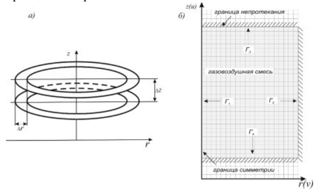
Рис. 2. Математическая постановка задачи: а) цилиндрический элемент расчетной сетки, б) расчетная сетка / The mathematical formulation of the problem: a) a cylindrical element of the computational grid, b) the estimated grid
