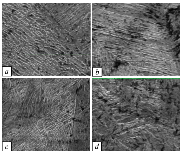
Рис.2. Растровые изображения бейнитной структуры ( \times 8050 ) металла швов ( a, c ) и участка перегрева ЗТВ ( b, d ) при лазерной сварке: V_{св} \sim 18 м/ч ( a, b ) и 50 м/ч ( c, d ); / Raster images of a bainite structure ( \times 8050 ) of the metal of welds ( a, c ) and the overheating area of HAZ ( b, d, f ) laser welding: V_{св} \sim 18 m / h ( a, b ) and 50 m / h ( c, d )
