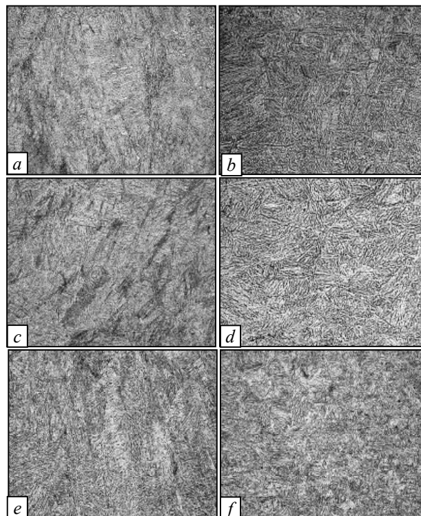
Рис. 1. Микроструктура металла (x500) швов (а, с, е) и участка перегрева ЗТВ (b, d, f) при лазерной сварке: V_{св} \sim 18 м/ч (а, b); 30 м/ч (с, d) и 50 м/ч (е, f); / The microstructure of the metal (x500) of welds (a, c, e) and the overheating area of HAZ (b, d, f) laser welding: V_{св} \sim 18 м / h (a, b); 30 м / h (c, d) and 72 м / h (e, f)
