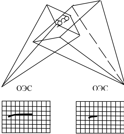
Рис. 1. Зависимость длины «следа» КО на регистрирующем элементе от размеров поля зрения ОЭС: – ОЭС1 – длина «следа» КО достаточная для селекции на фоне звезд по скорости; – ОЭС2 – длина «следа» КО недостаточная для селекции
