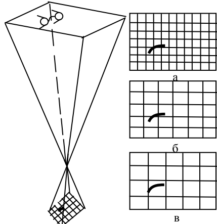
Рис. 2. Возможность селекции КО по длине «следа» в зависимости от линейных размеров элемента разложения фотоприемника: а – длина «следа» КО достаточная для селекции на фоне звезд по скорости; б, в – длина «следа» КО недостаточная для селекции
