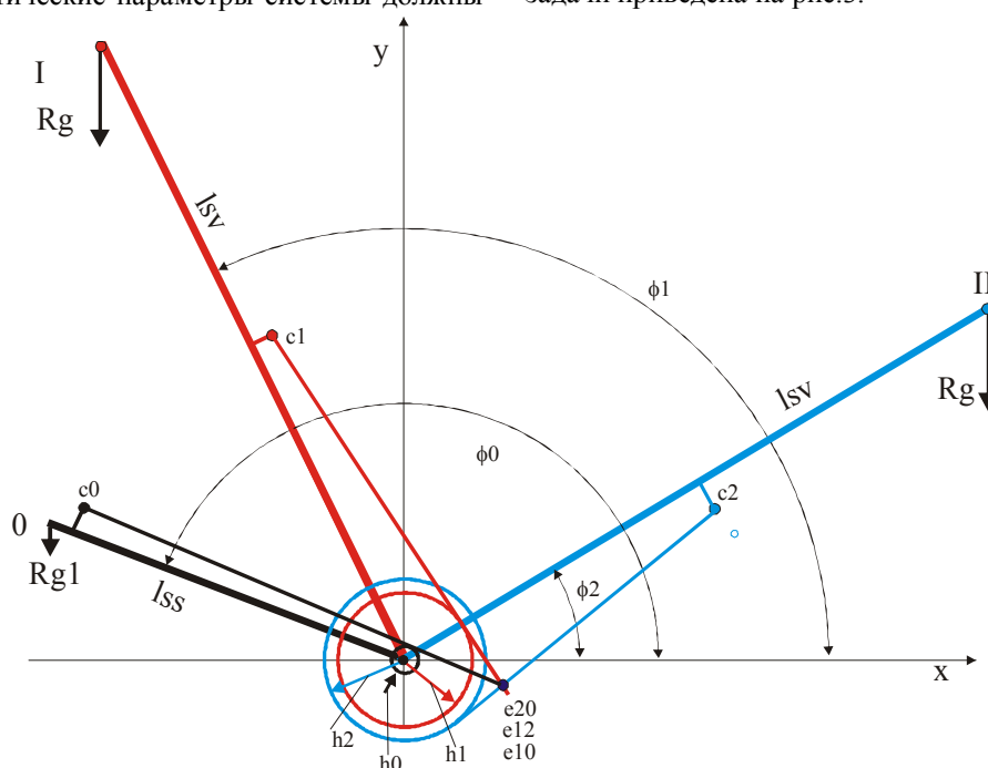
Рис. 3. Расчетная схема выбора параметров ГЦ и мест его крепления на СТ и на раме ТЗМ: R_g – вес груза; R_{g1} – сила веса от стрелы с вдвинутой секцией; c_0, c_1, c_2 – точки крепления гидравлического домкрата к стреле; e_{10}, e_{12}, e_{23} – точки крепления гидравлического домкрата к раме агрегата; h_0, h_1, h_2 – плечи гидравлического домкрата в положениях 0, I, II. Положения СТ: 0 – транспортное положение стрелы манипулятора, I – положение стрелы манипулятора при работе с грузом над ТЗМ, II – положение стрелы манипулятора при работе с грузом над подвижным агрегатом
