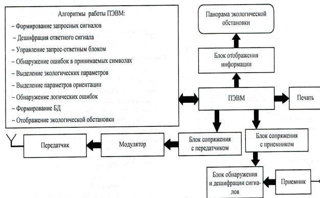
Рис. 2. Функциональная схема запрос-ответной автоматической системы экологического контроля
