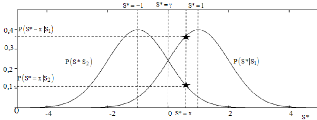
Рис. 1. Функции правдоподобия
