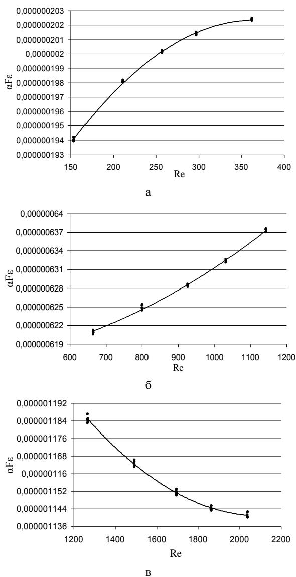
Рис. 2. Залежність коефіцієнта \alpha F_{\varepsilon} від числа Рейнольдса а – ЗП з m = 0,05 ; б – ЗП з m = 0,16 ; в – ЗП з m = 0,36
