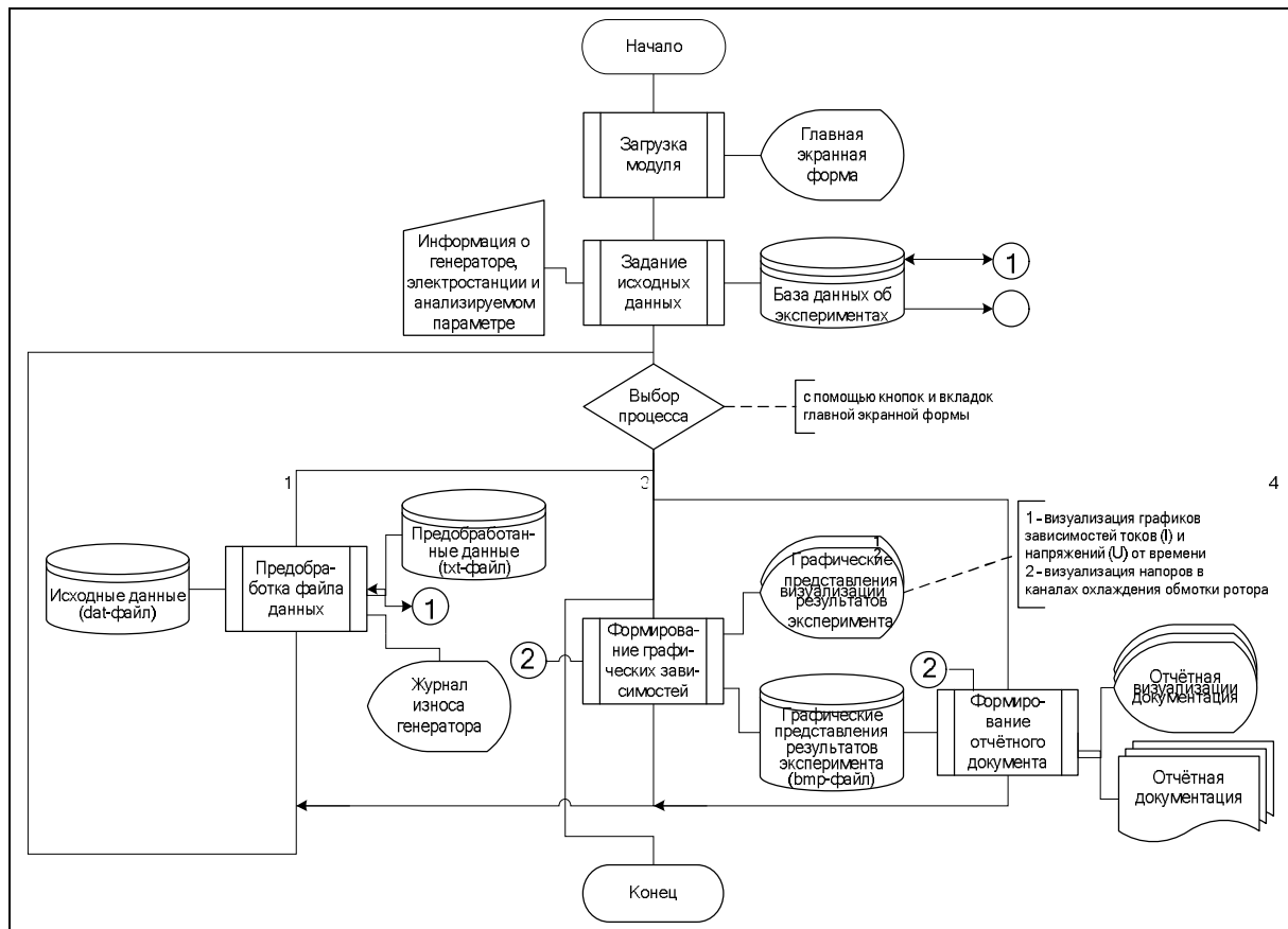
Рис. 2. Алгоритм обработки и визуального анализа данных о состоянии отдельных узлов турбогенератора
