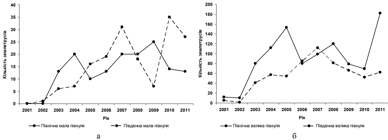
Рис. 4. Динаміка кількості землетрусів, що виникли у північній малій та великій (а) і південній малій та великій (б) піквулях за період 2001 – 2011 рр.
