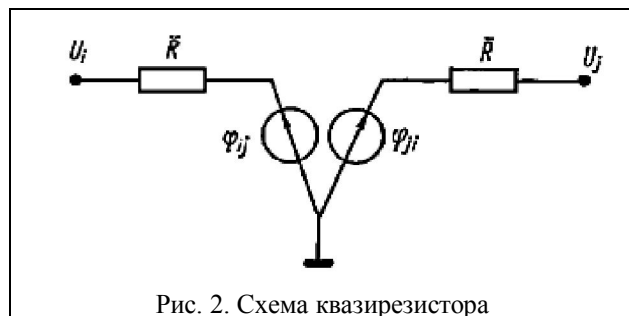
Рис. 2. Схема квазирезистора
