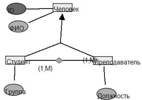
Рис. 4. Приклад ER-діаграми
