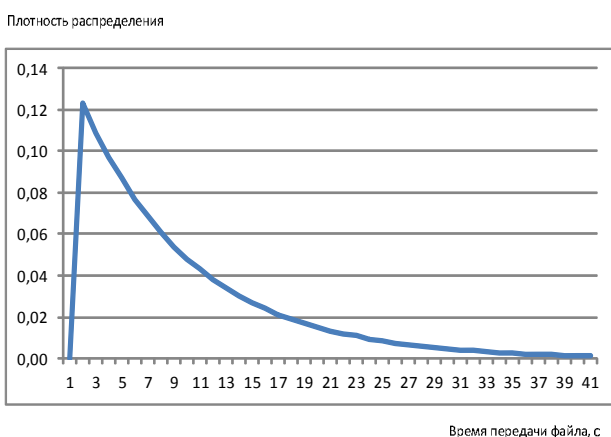
Рис. 3. Плотность распределения времени передачи метаданных в облачные антивирусные системы
