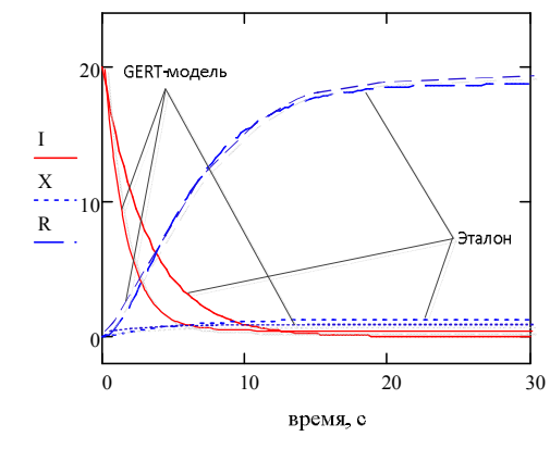
Рис. 4. Графики зависимости количества зараженных ( I ), выведенных из строя ( X ), и вылеченных (обладающих иммунитетом ( R )) объектов от времени функционирования информационно-телекоммуникационной сети
