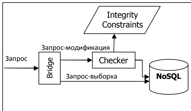
Рис. 3. Схема алгоритму перевірки обмежень цілісності
