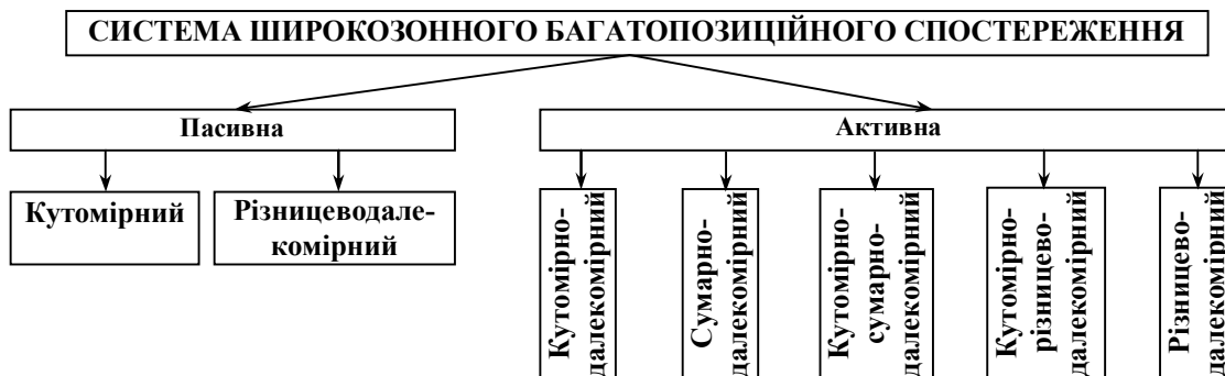
Рис. 1. Класифікація методів рішення координатної задачі системами ШБС
