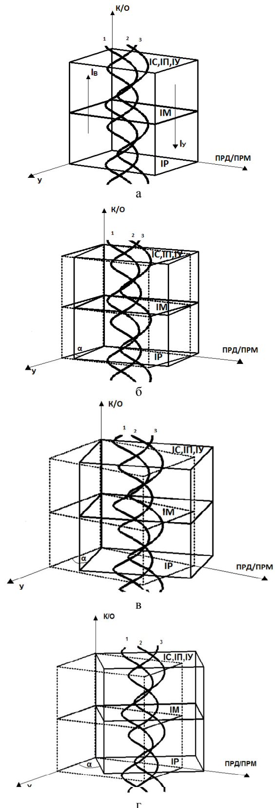
Рис. 3. Модель простору інформаційно-технічних станів БІСК у контексті гарантоздатності: а – працездатний (безпечний) стан – NORMA; б – частково працездатний (безпечний) стан – ALARM-1; в – непрацездатний (безпечний) стан – ALARM-2; г – непрацездатний небезпечний стан – AVARIA
