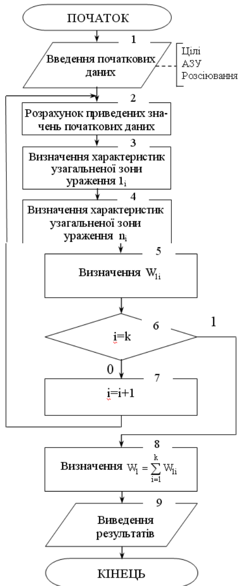
Рис. 3. Алгоритм визначення імовірності ураження одиночної цілі при застосуванні різнотипних АЗУ
