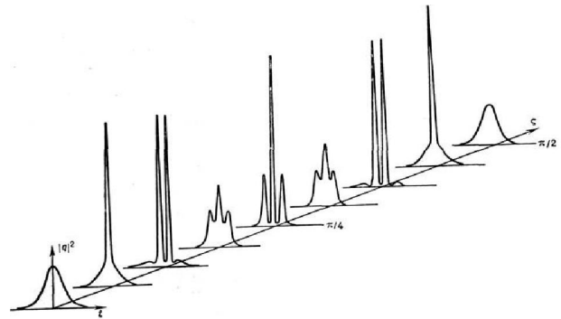
Рис. 1. Самоістиска N -солітонового імпульсу при нерезонансному самовпливові у волоконному світловоді ( N = 4 )
