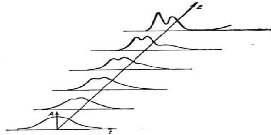
Рис. 2. Розбивка імпульсу на три імпульси при резонансному самовпливові
