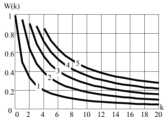
Рис. 1. Залежність ймовірності ураження РЛС - W(k) , від кількості випромінювачів-пасток, при послідовному пуску 1, 2, 3, 4, 5 ПРП відповідно
