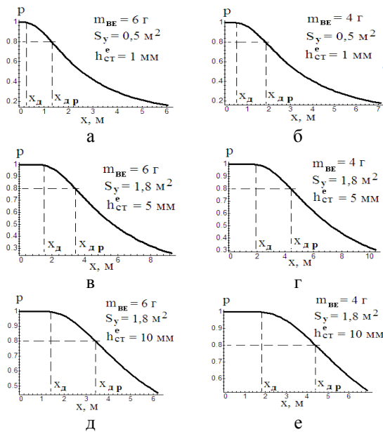
Рис. 2. Залежність значень імовірності ураження типових ЕО від відстані x від точки розриву ОФБЕ при різних масах ВЕ x_d – радіус області достовірних уражень ЕО; x_{dP} – радіус розширеної області достовірних уражень ЕО
