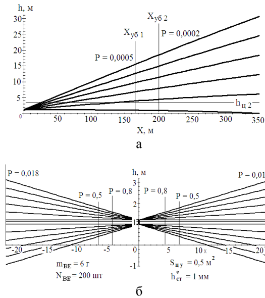
Рис. 1. Вертикальний перетин динамічного поля ВЕ при розриві ОФБЕ на висоті 1 м X_{y6 1} – убойча дальність ВЕ з масою 4 г; X_{y6 2} – убойча дальність ВЕ з масою 6 г (для незахищеної живої сили)
