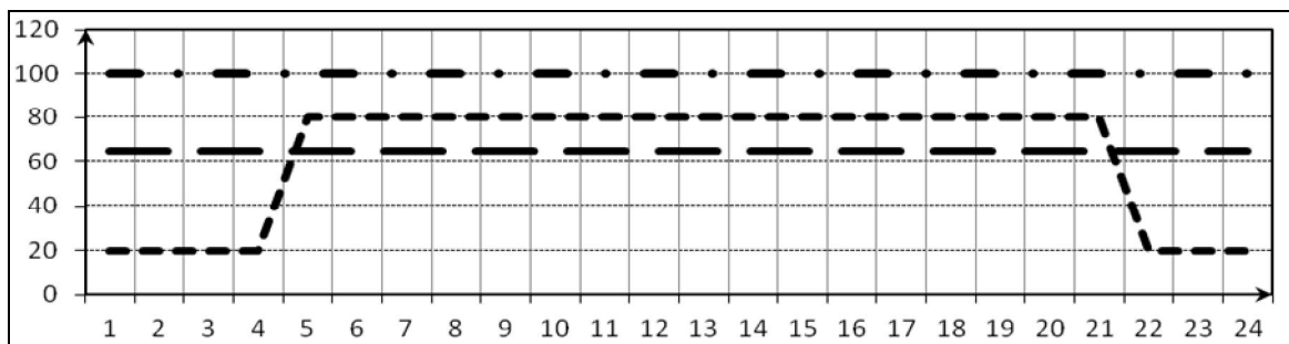
Рис. 1. Гармонограма зміни потужності у часі:
