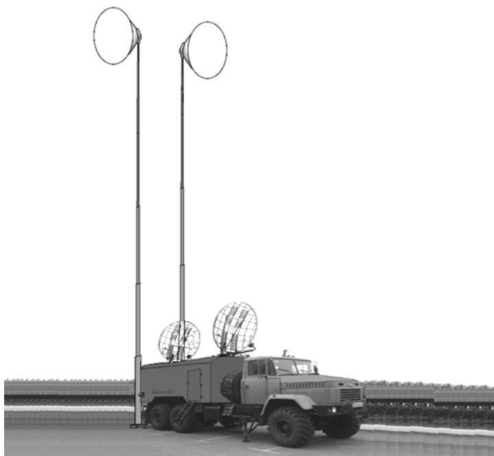
Рис. 2. Конструктив цифровой тропосферно-радиорелейной станции на базе тропосферных станций (Р-412, Р-417, Р-423-1)
