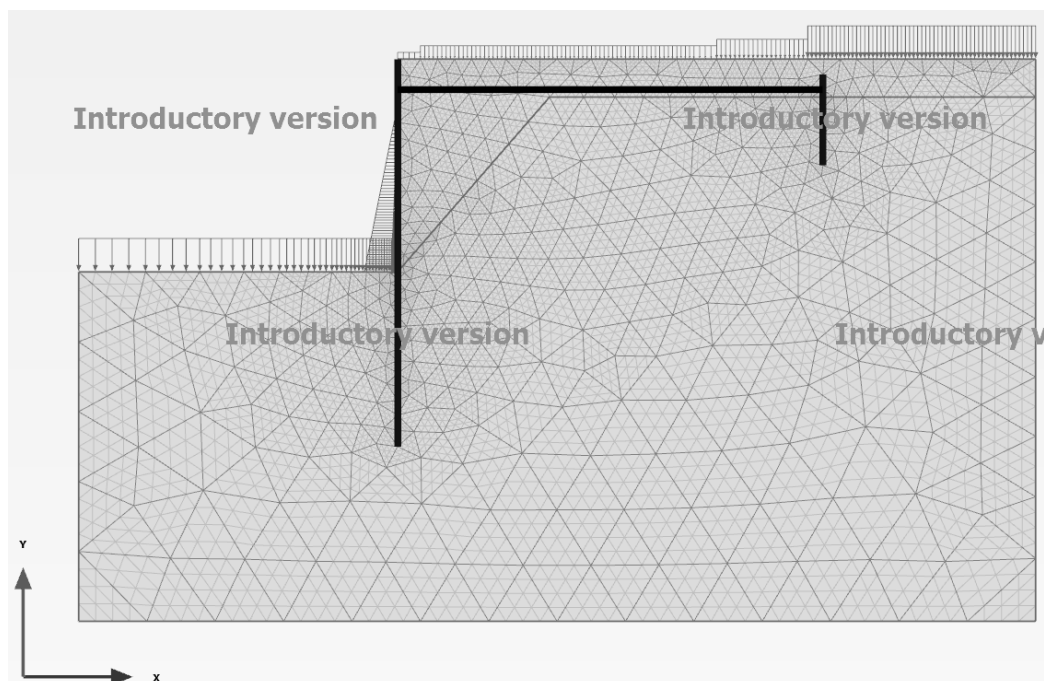
Рис.2. Розрахункова схема
