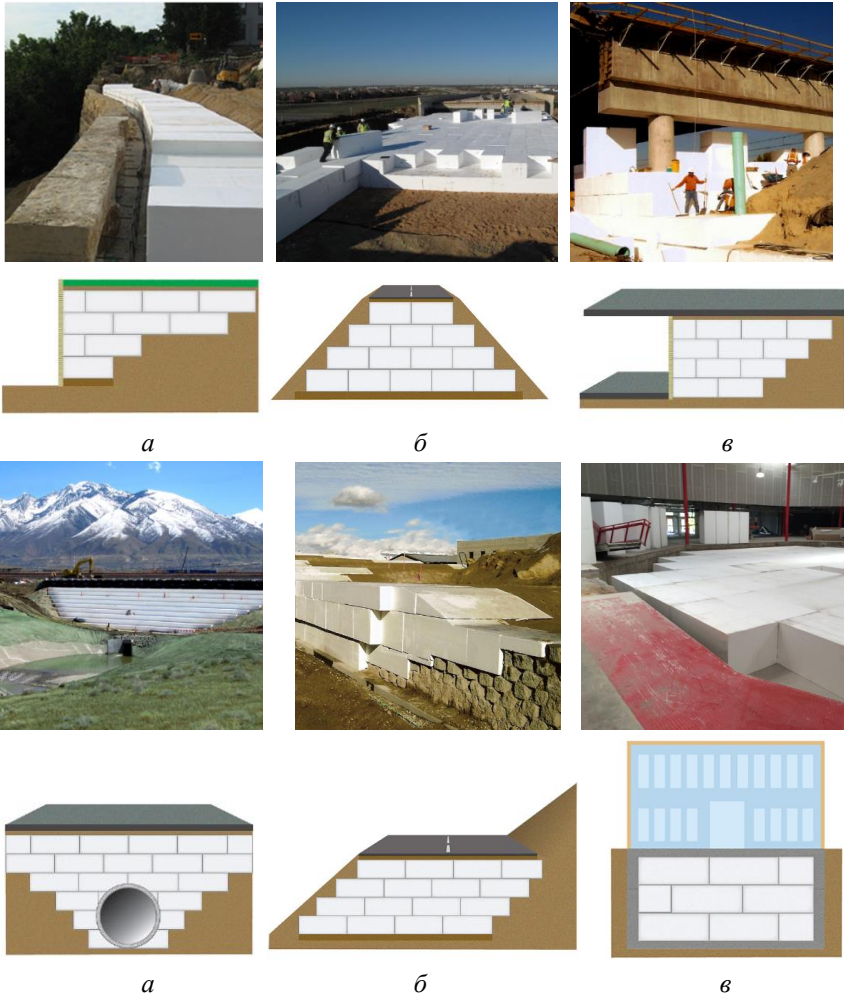
Рис. 1. Застосування блоків з геопіни для різних інженерних рішень [1]
