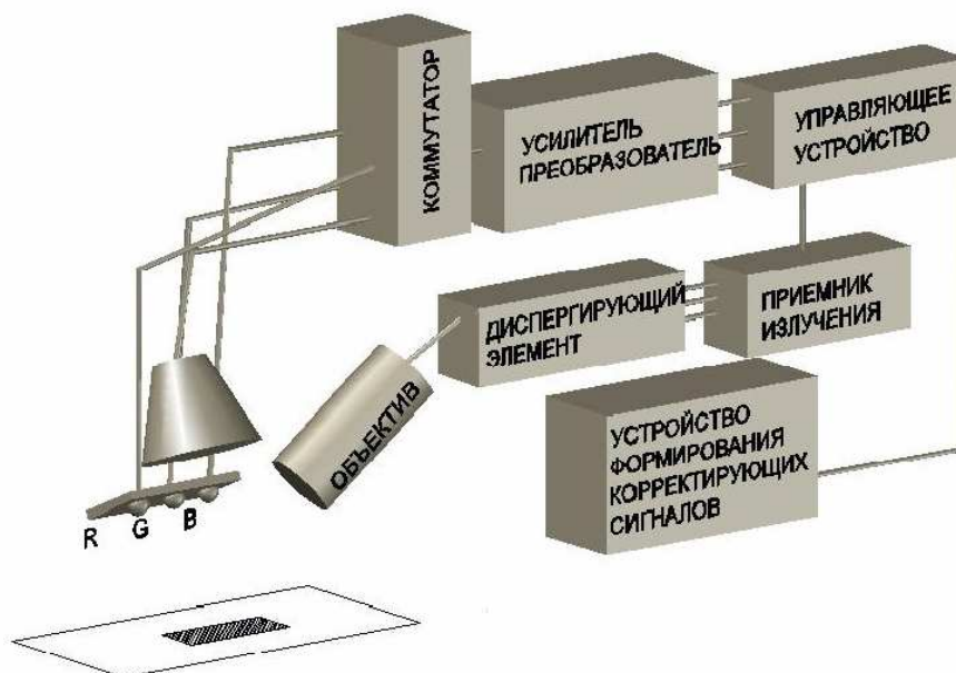
Рис.1 – Структурная схема яркостной и цветовой коррекции
