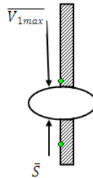
Рис. 2. Схема ударної взаємодії при защемленні зернівки в отворі решета при її русі вниз по поверхні решета
