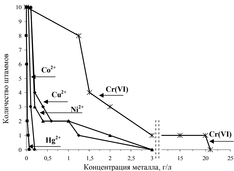
Рис. 2. Зависимость количества выживших штаммов микроорганизмов антарктических клифов от концентрации \text{Hg}^{2+} , \text{Co}^{2+} , \text{Ni}^{2+} , \text{Cu}^{2+} и Cr(VI) в среде NB.
