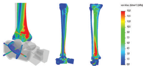
Рис. 11. Распределение напряжений на фиксирующих элементах модели импрессионного перелома пяточной кости, фиксированной винтами
