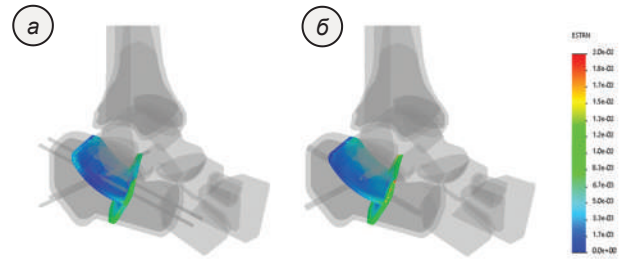
Рис. 13. Распределение относительных деформаций на фиксирующих элементах модели внутрикостного остеосинтеза импрессионного перелома пяточной кости спицами (а) и винтами (б)
