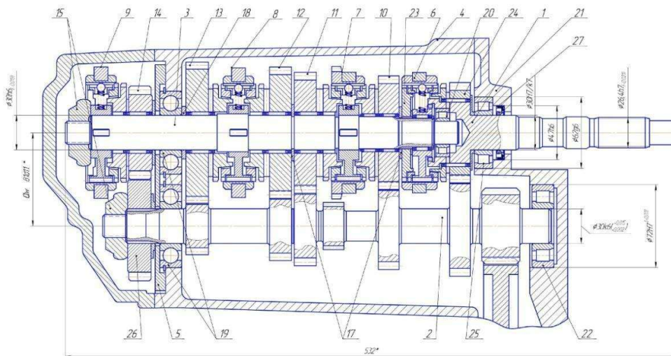
Рис. 2. Складальний креслення розробленої трьохвалної коробки передач:
