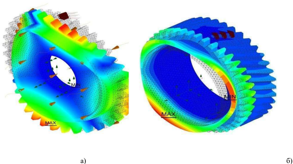
Рис. 9. 5-я форма власних коливань: а) шестерня постійного зачеплення; б) шестерня п'ятої передачі
