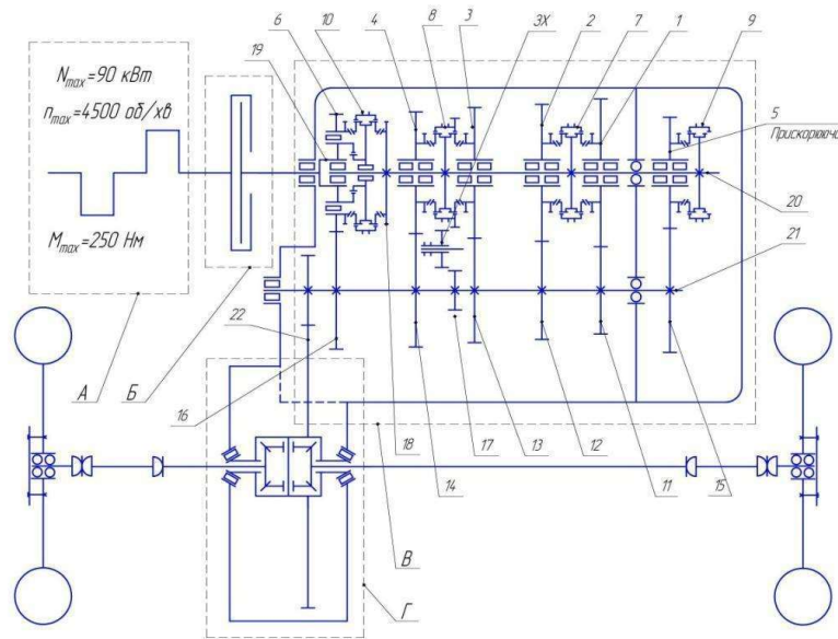
Рис. 1. Кінематична схема трансмісії автомобіля з поперечним розташуванням двигуна та розробленою трьохвалною коробкою передач:
