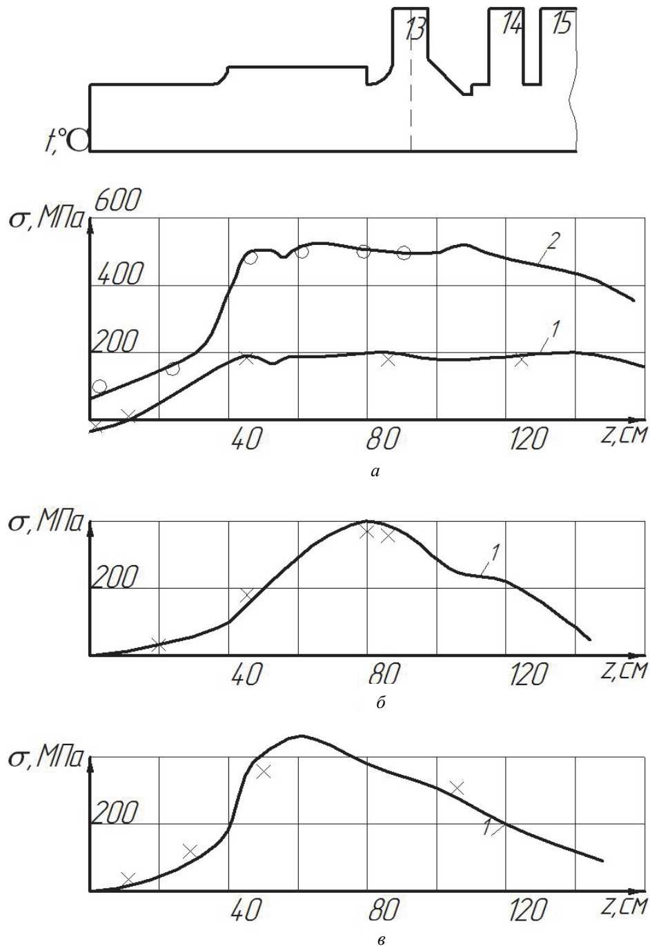
Рис. 1 – Сравнение НДС (кривая 1) и ТС (кривая 2) авторов [5] с расчётными данными при 3D моделировании: а – при пуске из ХС; б – НС-1; в – ГС; о – ТС РСД; × – НДС РСД
