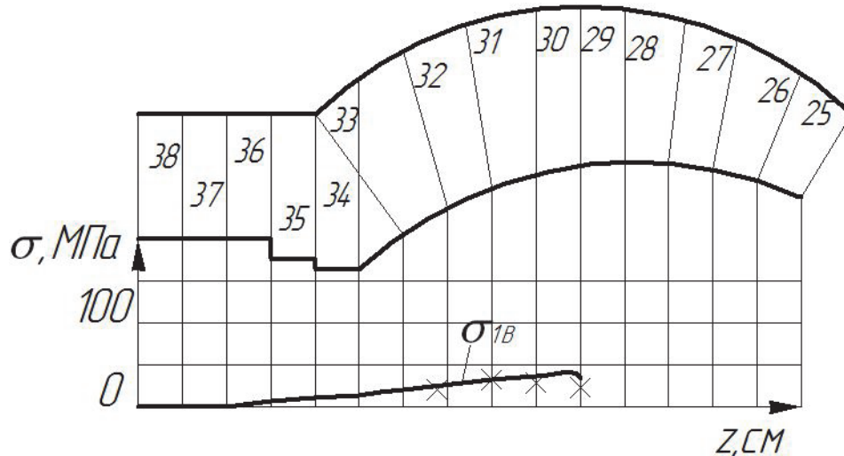
Рис. 3 – Сопоставление НДС ( \sigma_{1v} ) авторов [7] с расчётными данными при 3D моделировании АСК ЦВД: \sigma_{1v} , × – НДС внутренней поверхности АСК ЦВД
