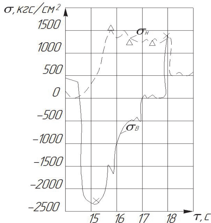
Рис. 2 – Сравнение НДС ( \sigma_n , \sigma_b ) авторов [6] при пуске после 48 часов простоя с расчётными данными при 3D моделировании:
