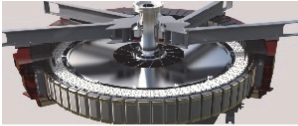
Рис. 1 – Вертикальний гідрогенератор конструкції Andritz
