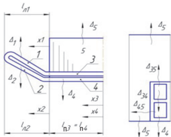
Рис. 4 – Схема расчётной модели двухслойной обмотки статора электрической машины
