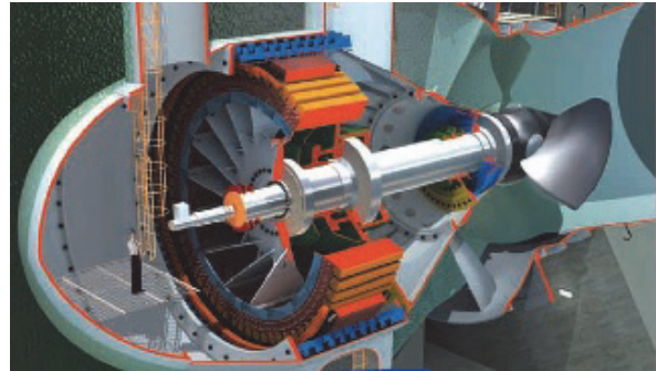
Рис. 3 – Капсульний гідрогенератор
