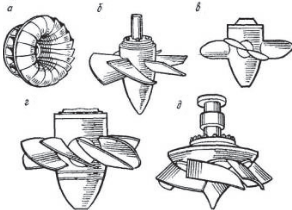
Рис. 2 – Обицїй вид робочих колес реактивних турбін: а – радіально-осева; б – пропеллерна; в – поворотнo-лопастна; г – двохперова, діагональна
