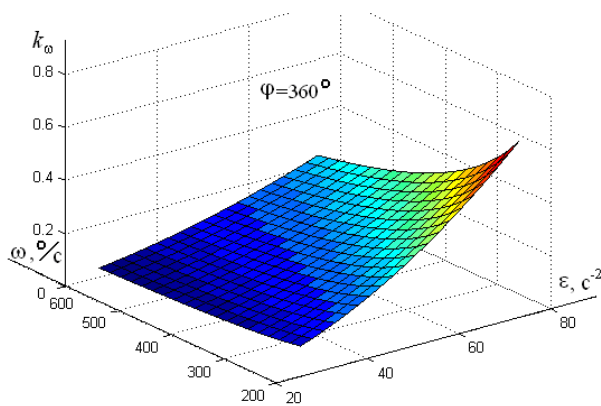
Рисунок 1 – Диаграмма критерия быстродействия для промышленных роботов легкой грузоподъемности при \varphi=360^\circ , табл. 1
