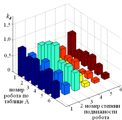
Рисунок 3 – Критерии динамичности по степеням подвижности промышленных роботов легкой грузоподъемности, табл. 1
