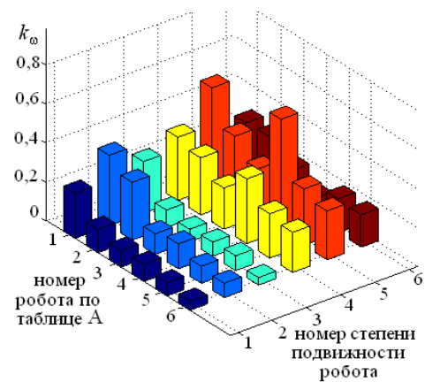
Рисунок 2 – Диаграмма критериев быстродействия по степеням подвижности промышленных роботов легкой грузоподъемности, табл. 1
