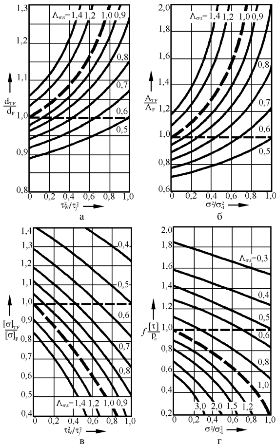
Рисунок 1 – Основные решения задачи проектирования силовых систем: а – определение диаметра вала; б – определение площади контакта; в – выбор материала; г – определение коэффициента трения
