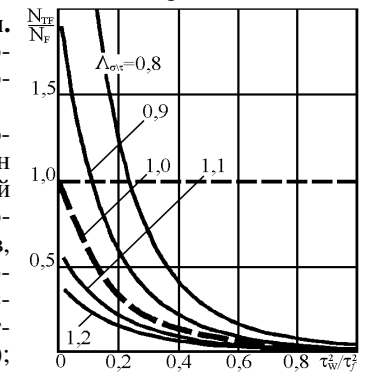
Рисунок 2 – Сравнение результатов ресурсного проектирования силовых систем ( m=12 )
