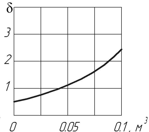
Рис.3 – Залежність декременту коливань від величини ємності додаткового резервуару
